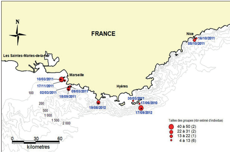
Figure 1. Localisation des groupes de grands dauphins Tursiops truncatus photo-identifiés durant l'étude (2011 et début 2012) et date des observations. Quatre tailles de groupe sont représentées par des cercles rouges de diamètre croissant en fonction du nombre estimé d'individus ; le nombre de groupes identifiés dans chaque catégorie est indiqué entre parenthèse. Chiffres noirs : isobathes (en m).
